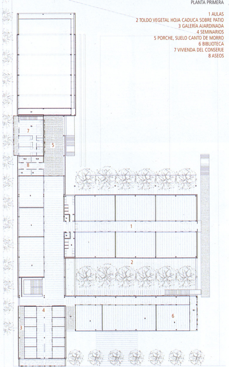
PLANTA PRIMERA
