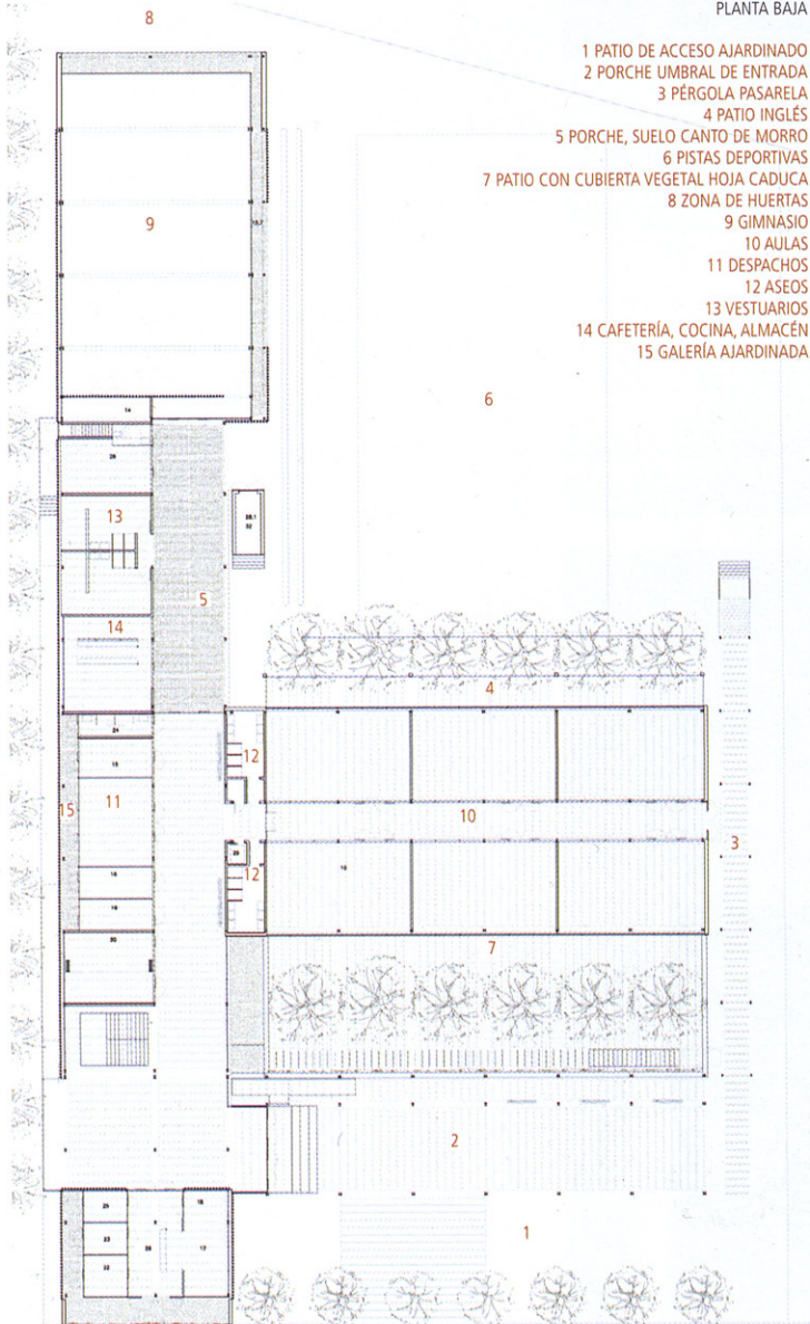
PLANTA BAJA
